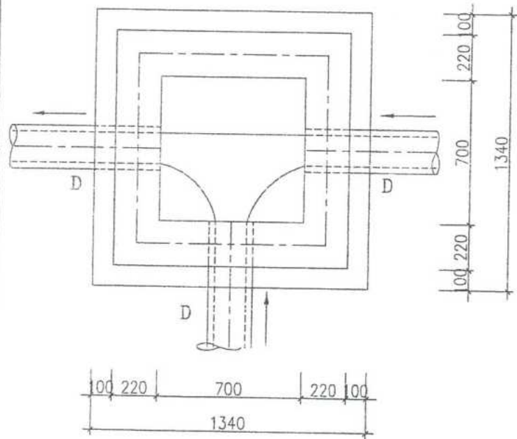
THÉP ĐÁY 1/10
