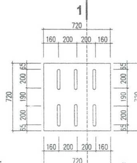
CHI TIẾT RĂNG KÍN TỶ LỆ 1:25
