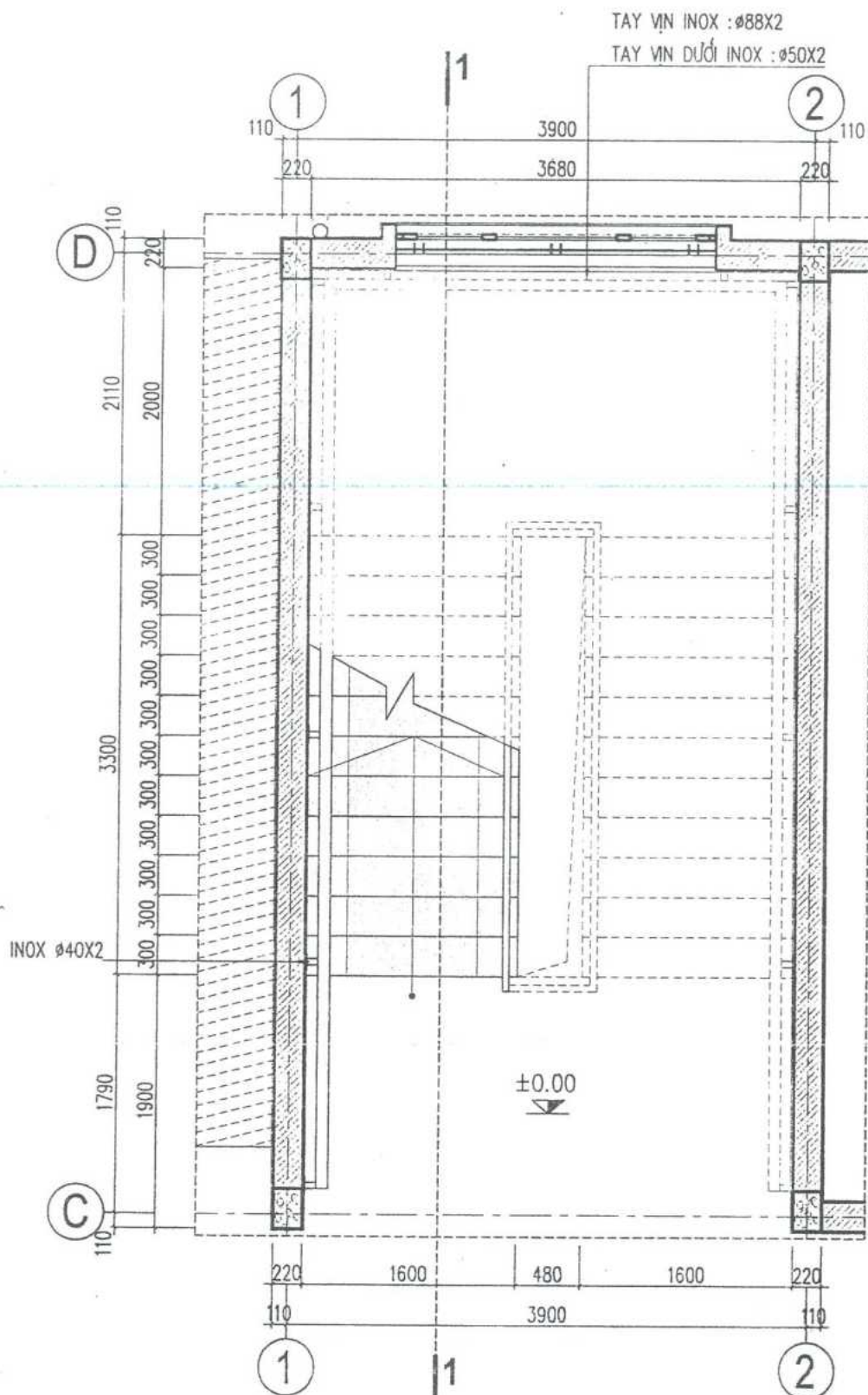
CHI TIẾT TH1 TỶ LỆ: 1/50 KT-04
