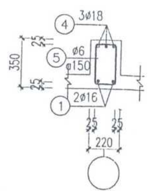
CẮT 11-11
