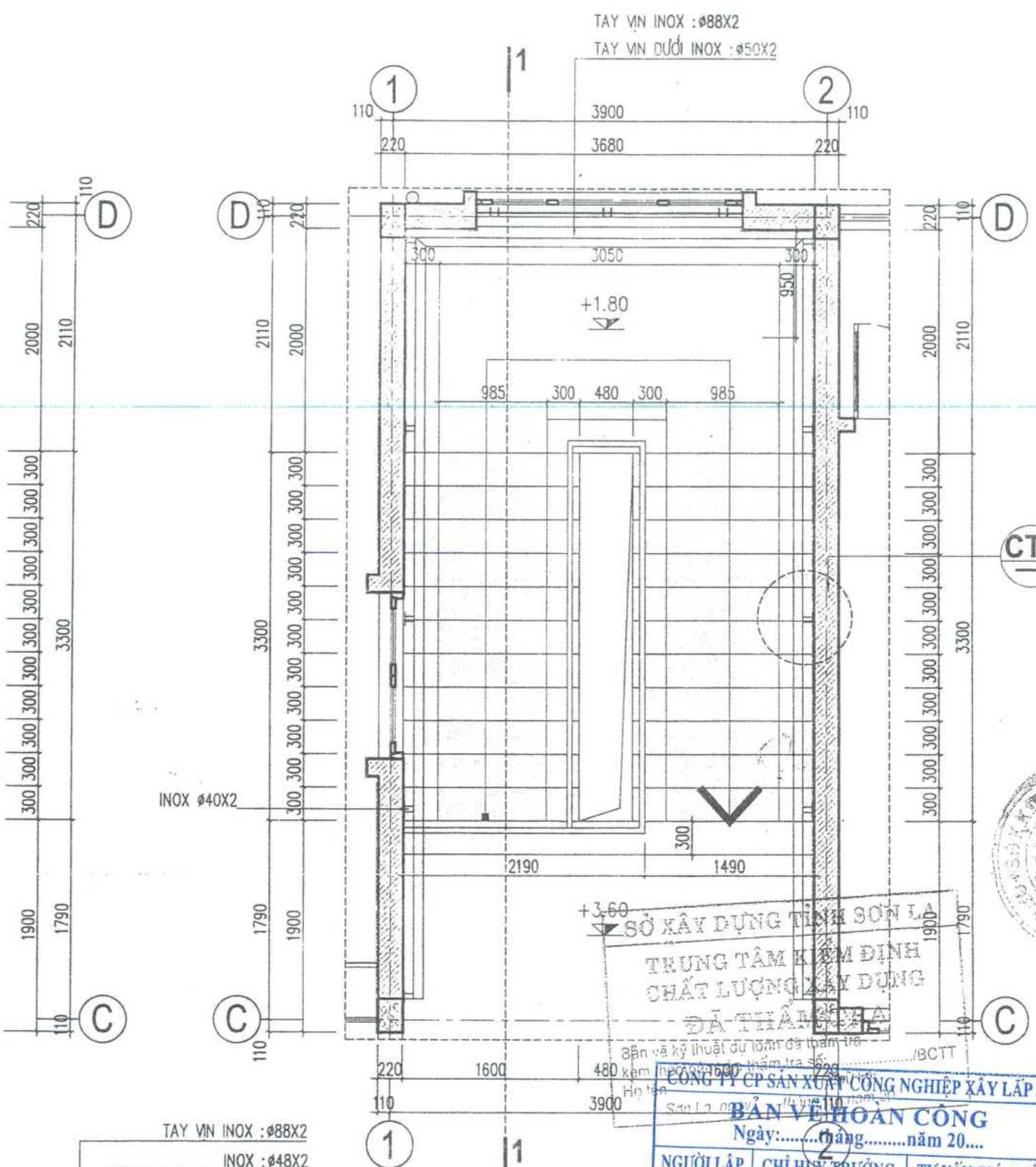
CHI TIẾT TH2 TỶ LỆ: 1/50 NGUYỄN VĂN NGUYỄN, NGUYỄN VĂN TIẾN, LÊ VĂN DƯƠNG
