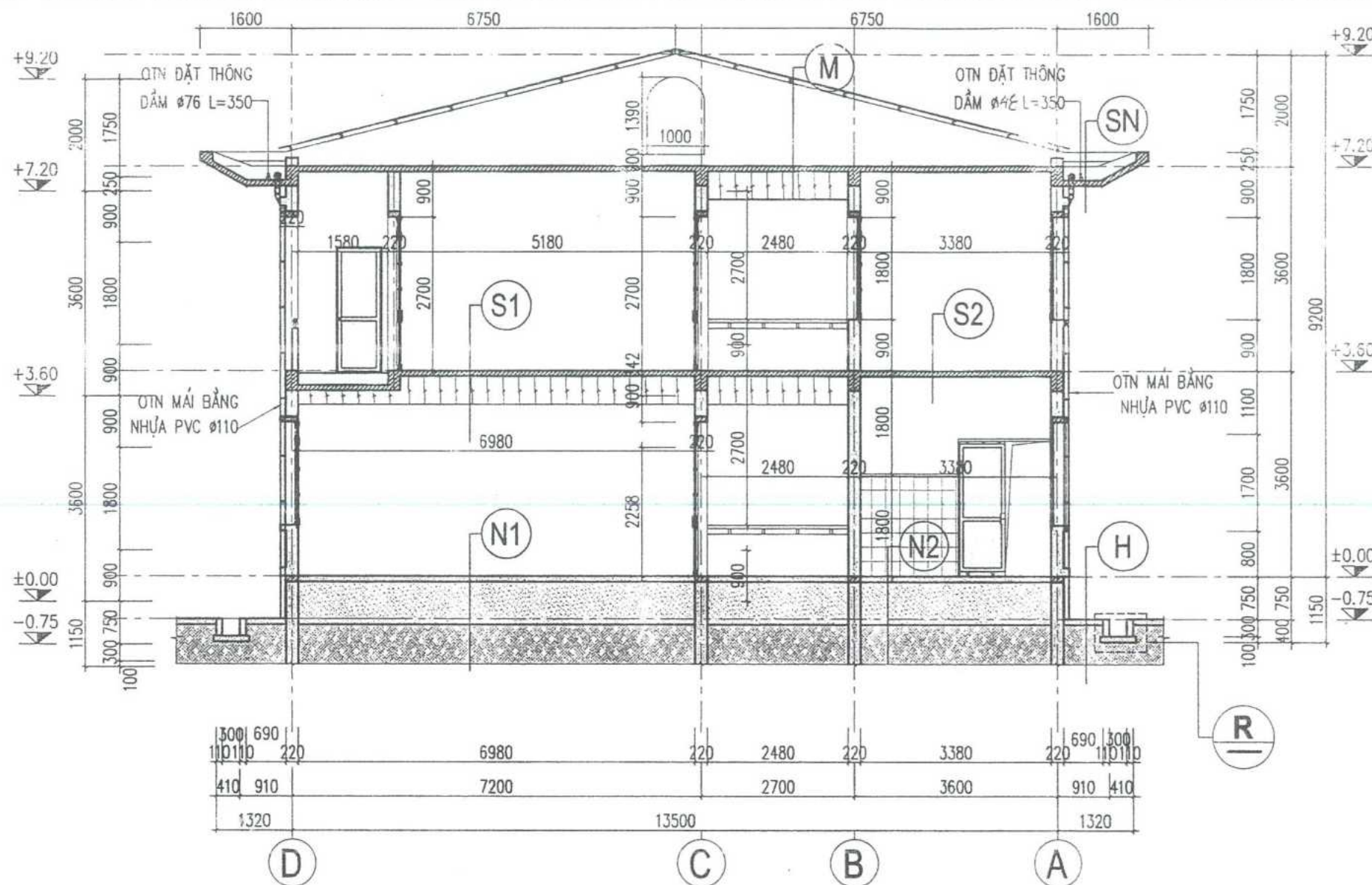
MẶT CẮT A-A TỶ LỆ 1:50
