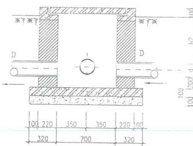
MẶT CẮT 1-1 1/20
