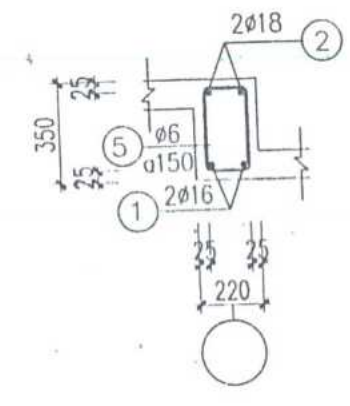
CẮT 9-9
