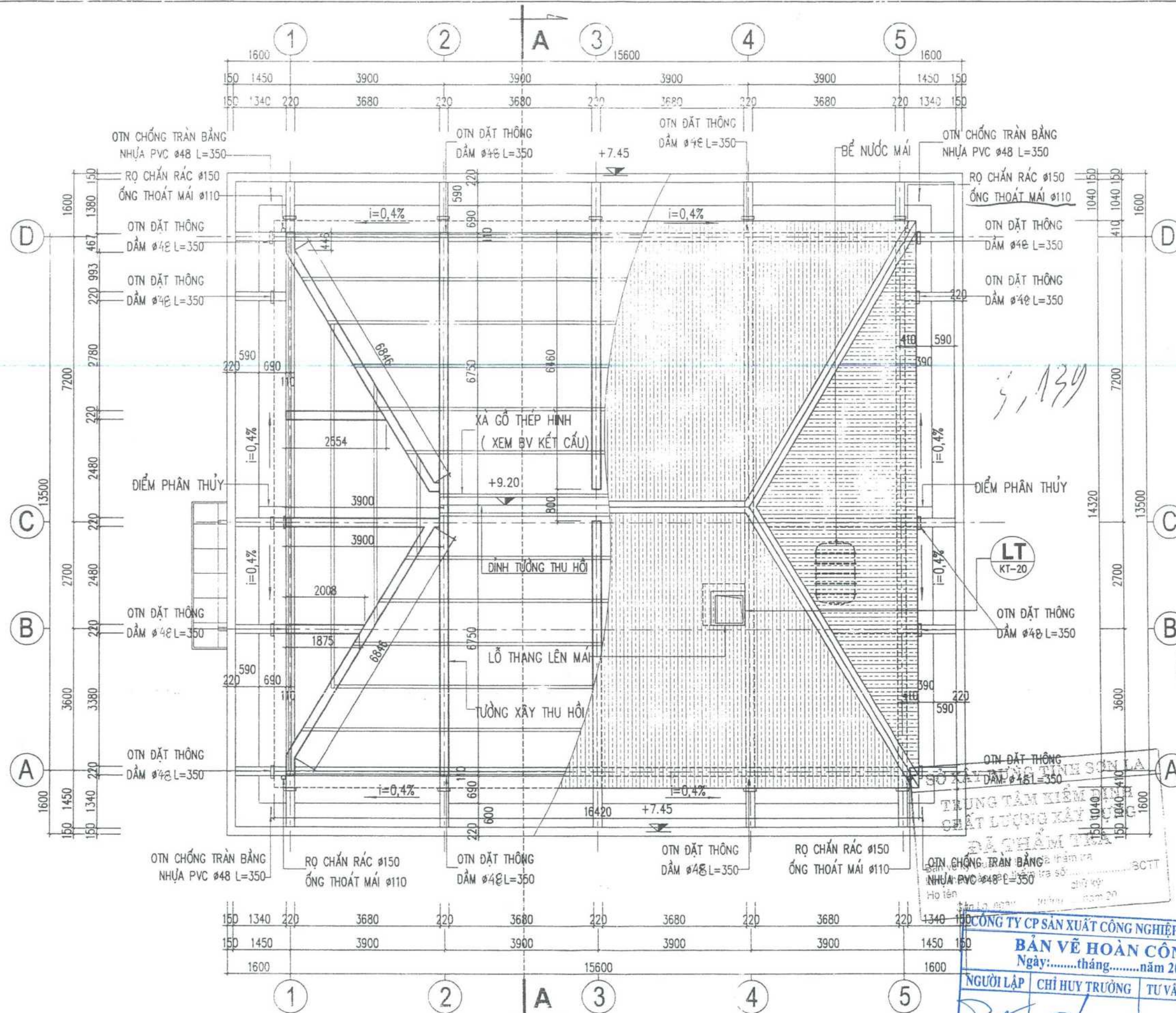
MẶT BẰNG MÁI TỶ LỆ 1:100
