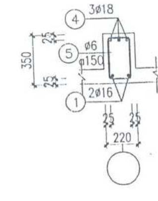
CẮT 11-11
