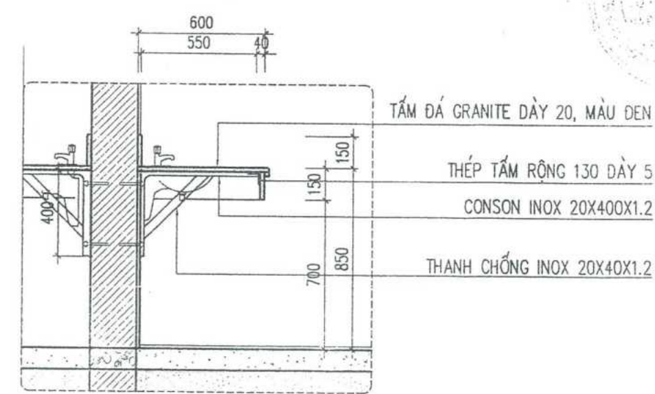
CHI TIẾT CHẬU RỬA TỶ LỆ 1:10
