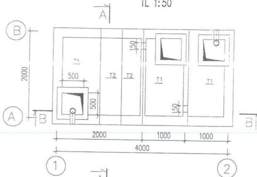
MẶT BẰNG BỂ TỰ HOẠI TL 1:50
