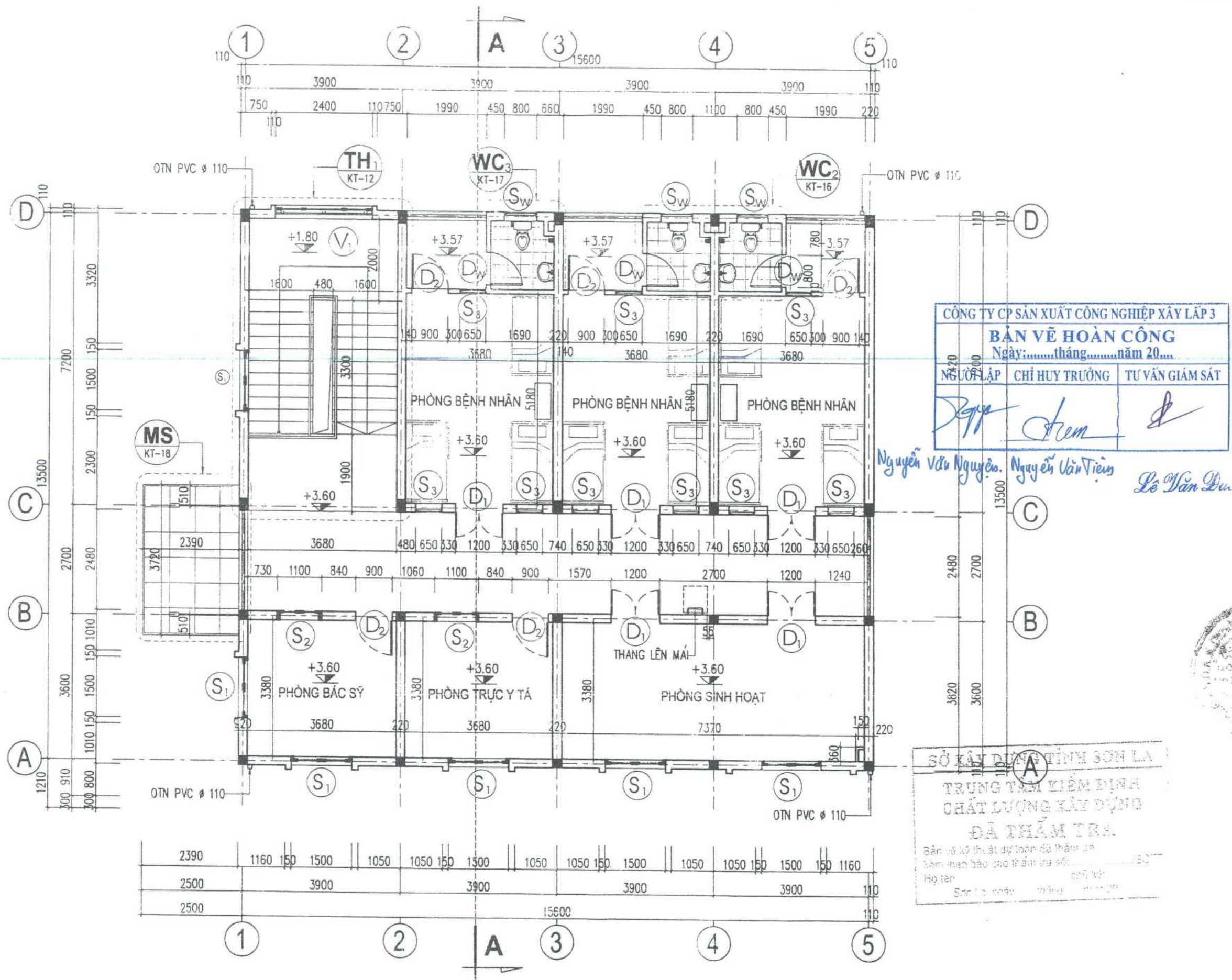
MẶT BẰNG TẦNG 2 TỶ LỆ 1:100
