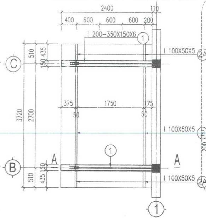
MẶT BẰNG KẾT CẤU KHUNG SÀN 1
