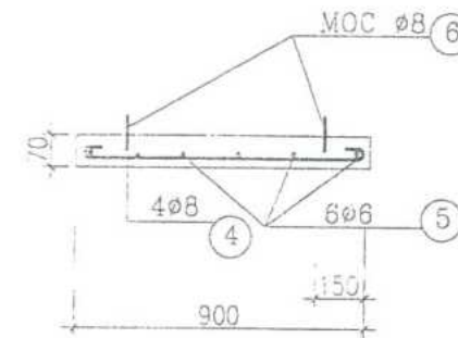
TẦM ĐÀN 1/10
