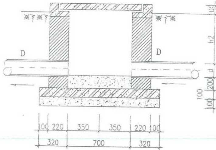
MẶT CẮT 2-2 1/20
