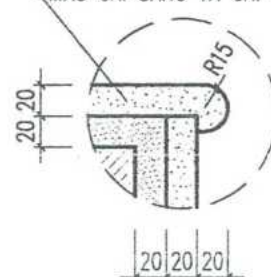
CHI TIẾT MŨI BẬC TỶ LỆ: 1/5
