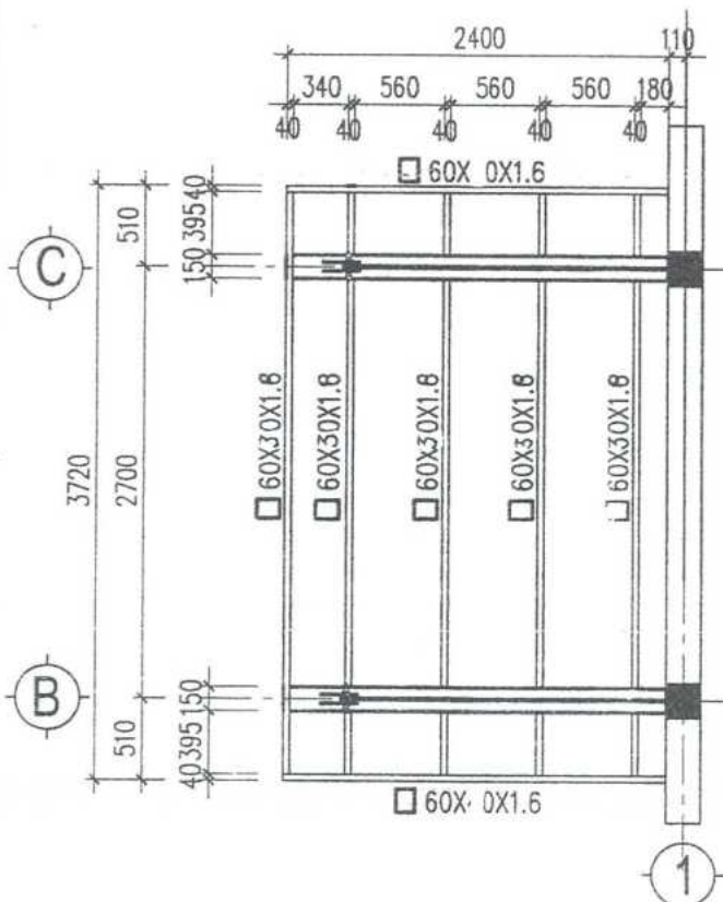
MẶT BẰNG XÀ GỖ LỚP DƯỚI
