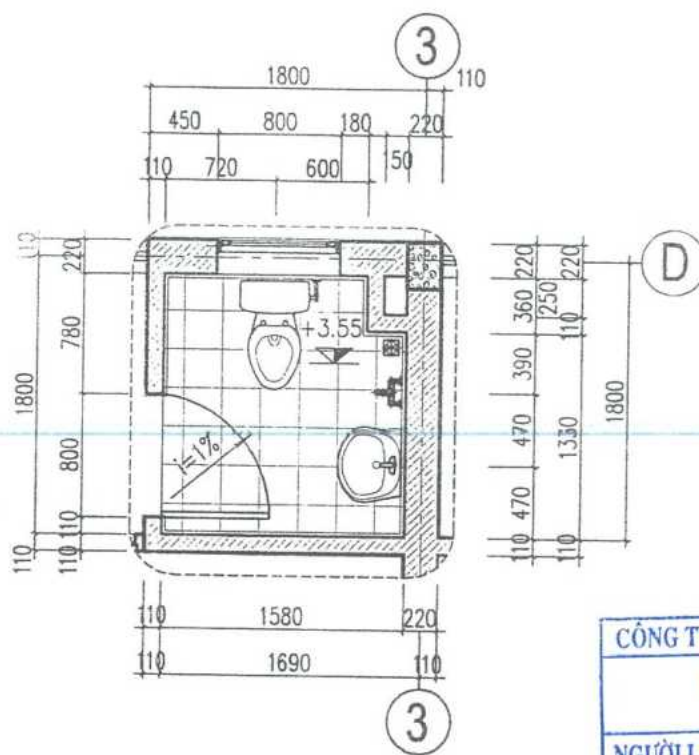
CHI TIẾT TỶ LỆ: 1/25
