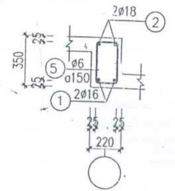
CẮT 9-9
