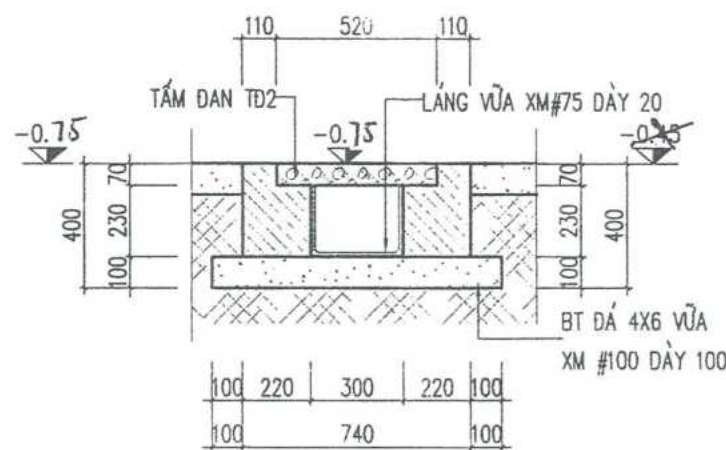
CHI TIẾT RĂNG KÍN TỶ LỆ 1:25
