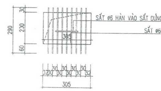
GHỊ CHẮN RÁC (TỶ LỆ: 1/10)
