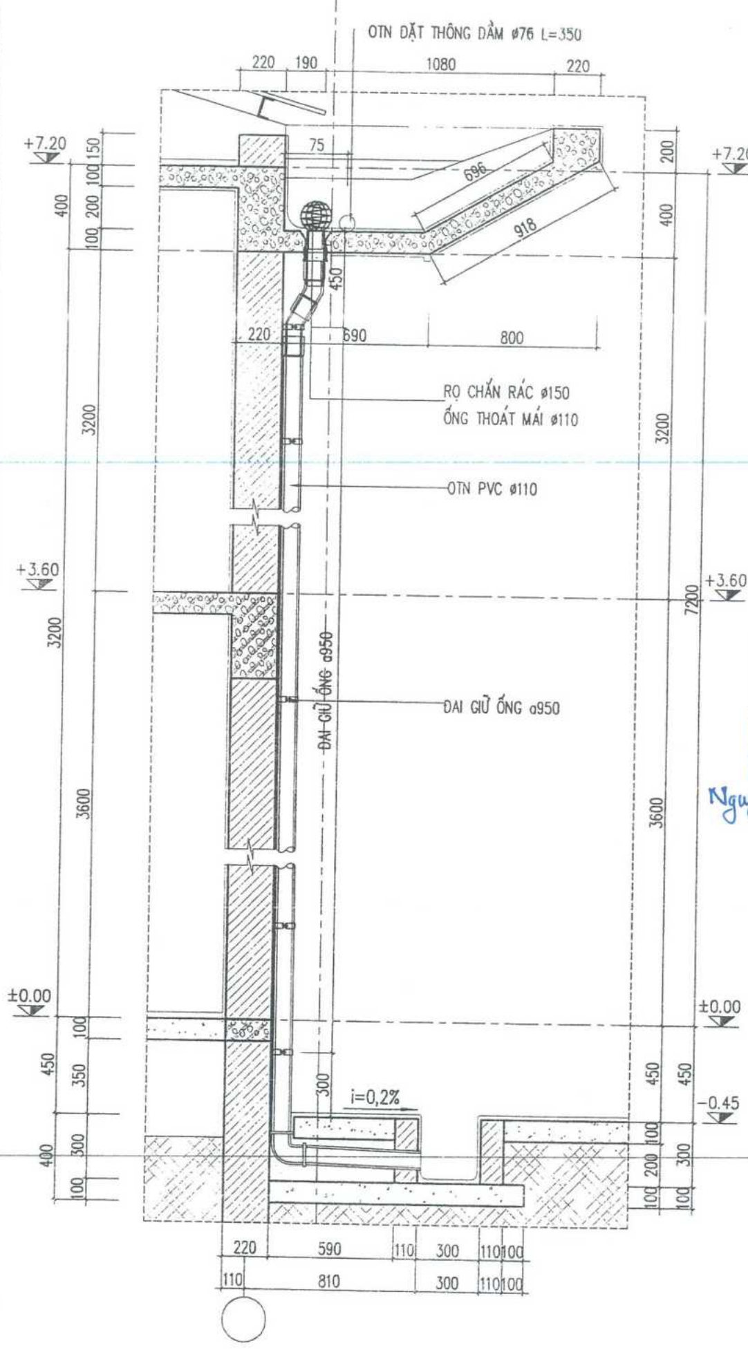
CHI TIẾT THOÁT NƯỚC MÁI (TỶ LỆ: 1/25)
