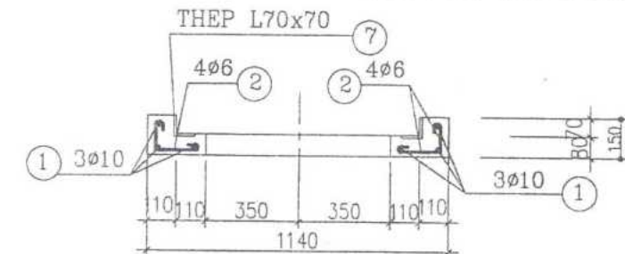
THÉP GIÀNG G1 1/10
