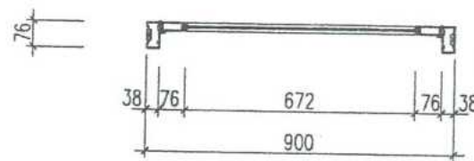
CẮT 1-1
