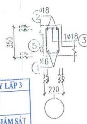
CẮT 10-10
