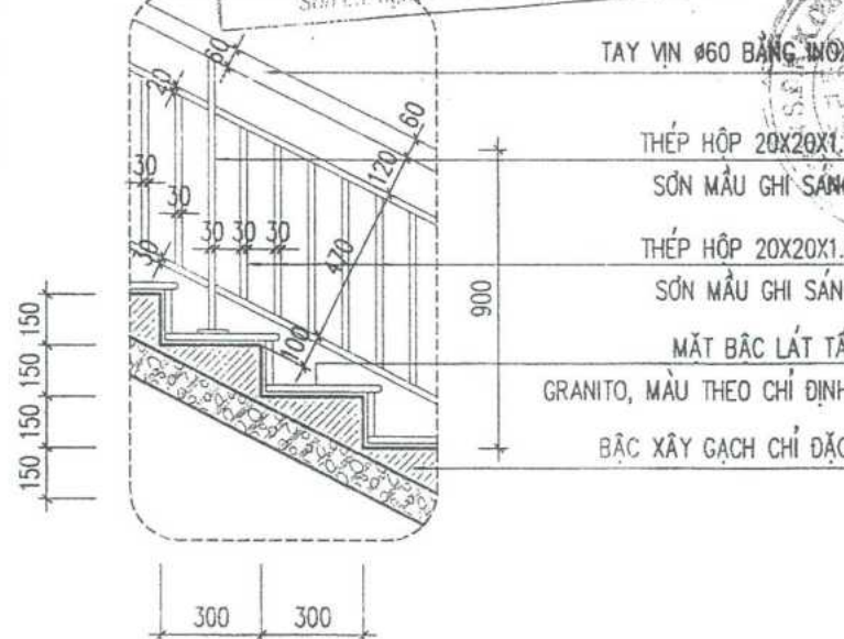
CHI TIẾT 1 (TỶ LỆ: 1/25)
