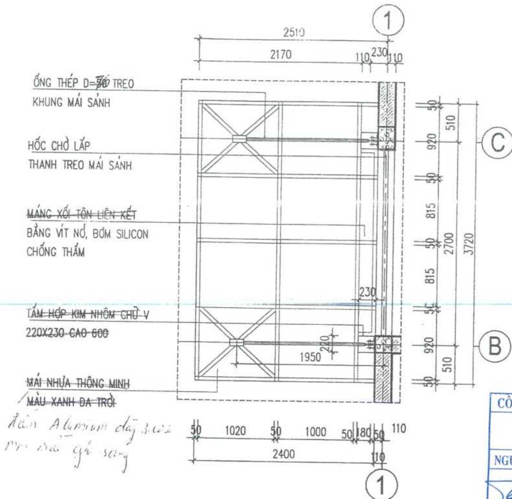
MẶT BẰNG MÁI SÁNH tỷ lệ : 1 / 50
