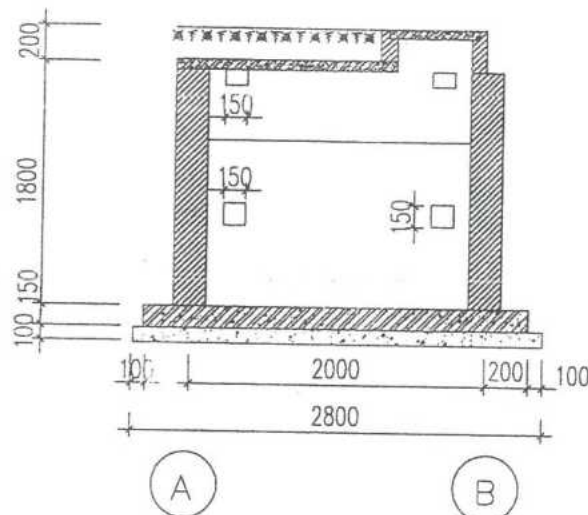
MẶT CẮT A-A TL 1:50
