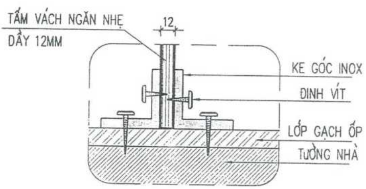
CHI TIẾT (TỶ LỆ: 1/4)
