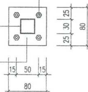
CHI TIẾT BẢN MÃ TỶ LỆ: 1/5
