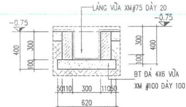
CHI TIẾT R TỶ LỆ: 1/25
