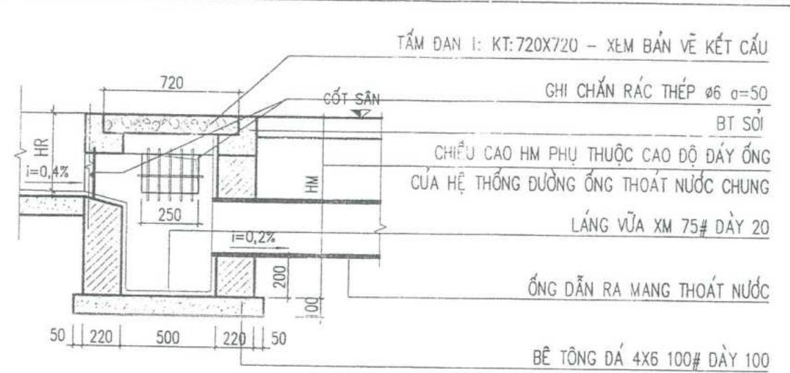
CẮT 1-1
