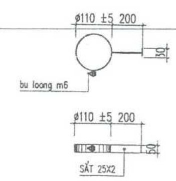
ĐẠI THÉP GIỮ ỚNG (TỶ LỆ: 1/10)
