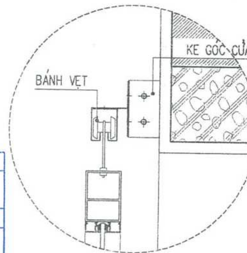
CHI TIẾT
