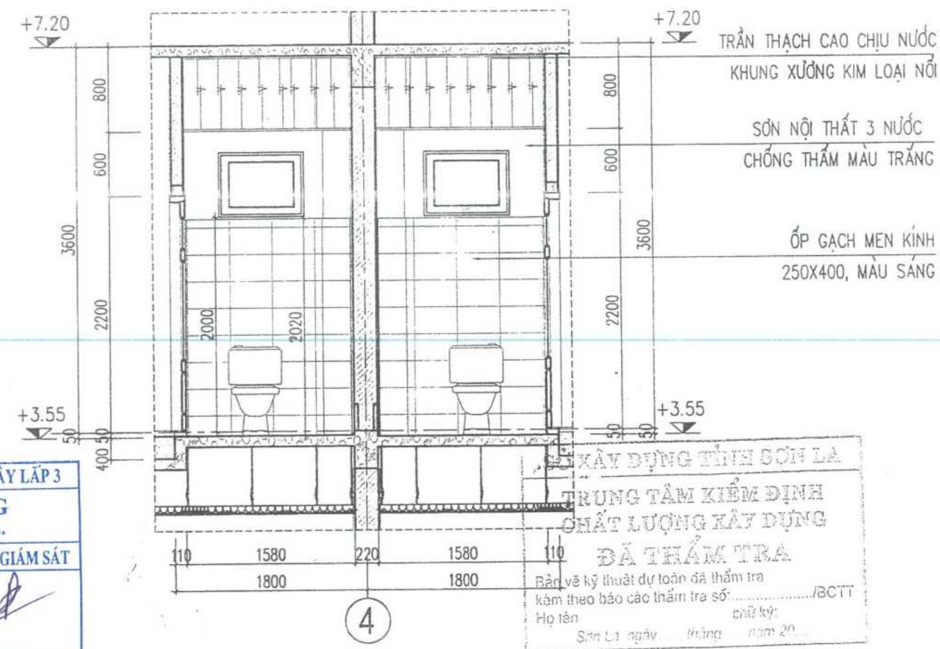
CẮT 3-3 TỶ LỆ 1:50
