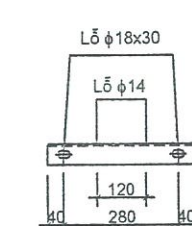
⑤ Thanh bắt ống TĐ CD
