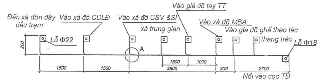
DÂY NỐI ĐẤT GIÀN TRAM (THÉP PHI10)
