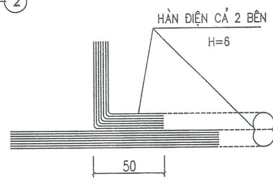
CHI TIẾT B
