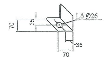
2 Tấm ốp
