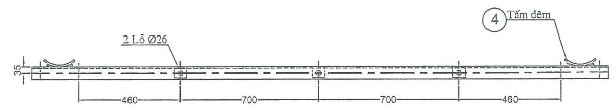
1 Thanh xà
