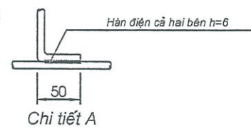
DÂY NỐI ĐẤT GIÀN TRAM (THÉP PHI10)
