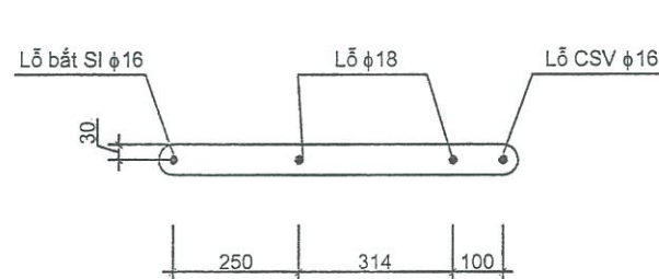
② Thanh bắt CSV và SI
