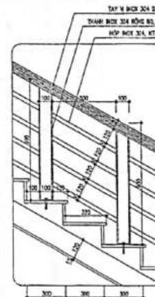
CHI TIẾT BẬC THANG
