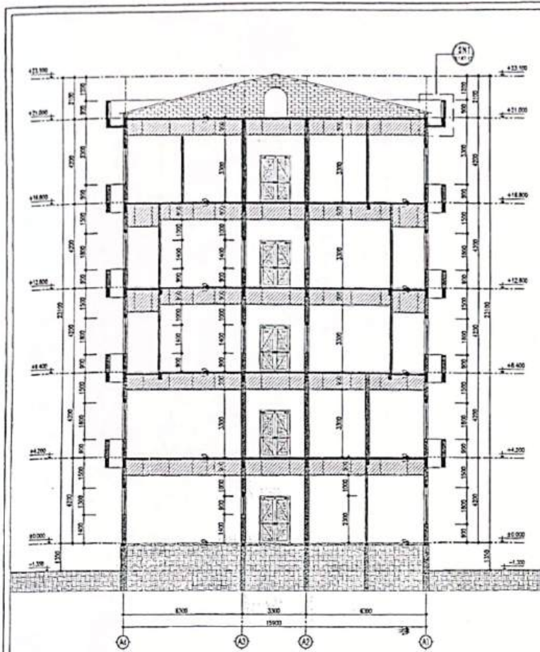
MẶT CẮT 3-3
