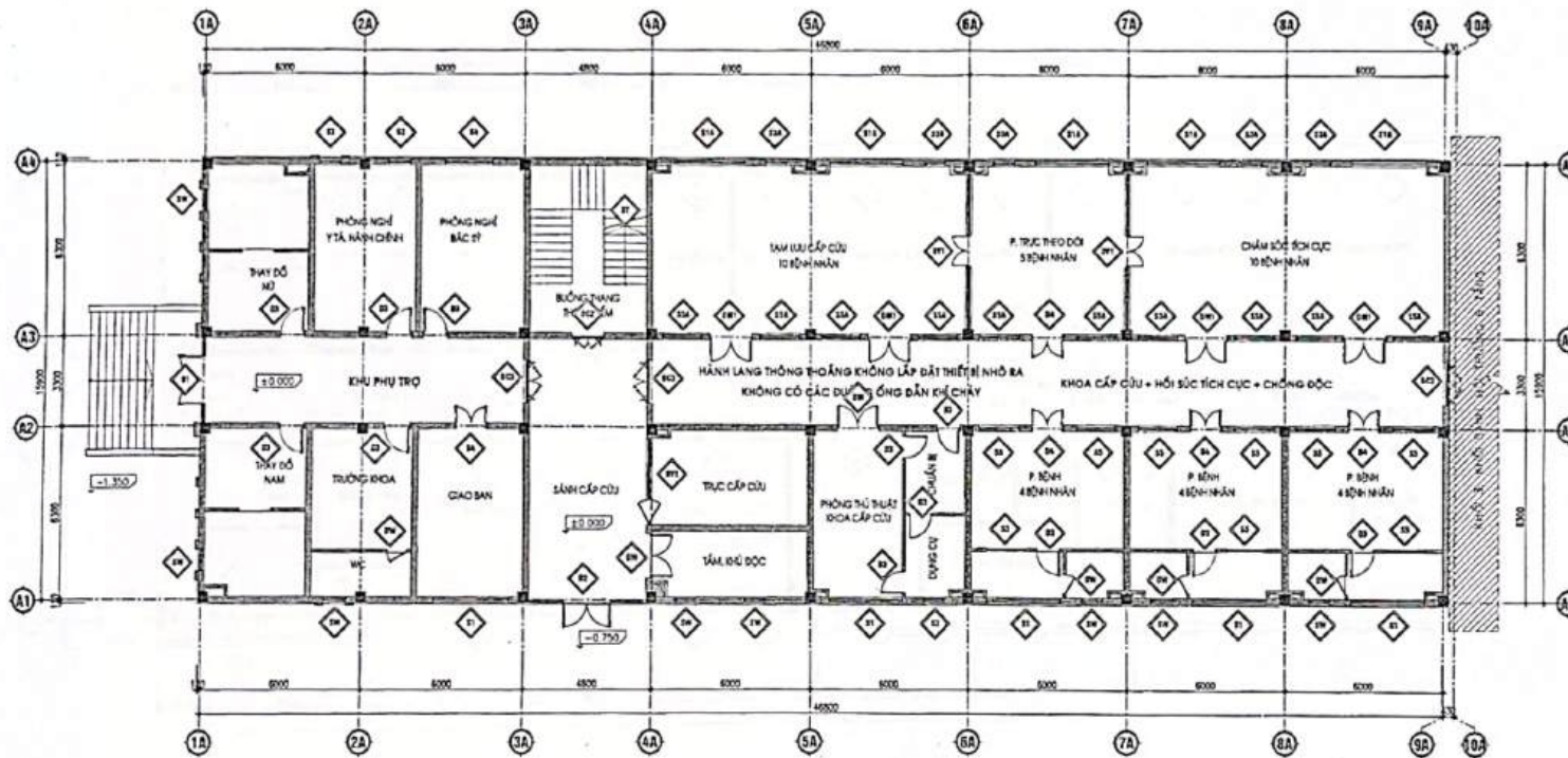
MẶT BẰNG ĐỊNH VỊ CỦA TẦNG 1
