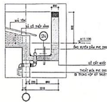
CHI TIẾT SÊ NÔ SN1
