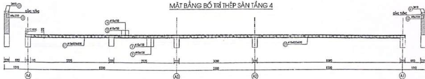
MẶT BẰNG BỐ TRÍ THÉP SÀN TẦNG 4
