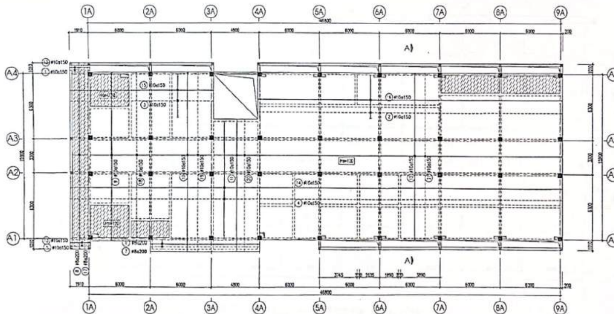
MẶT BẰNG BỐ TRÍ THÉP SÀN TẦNG 5
