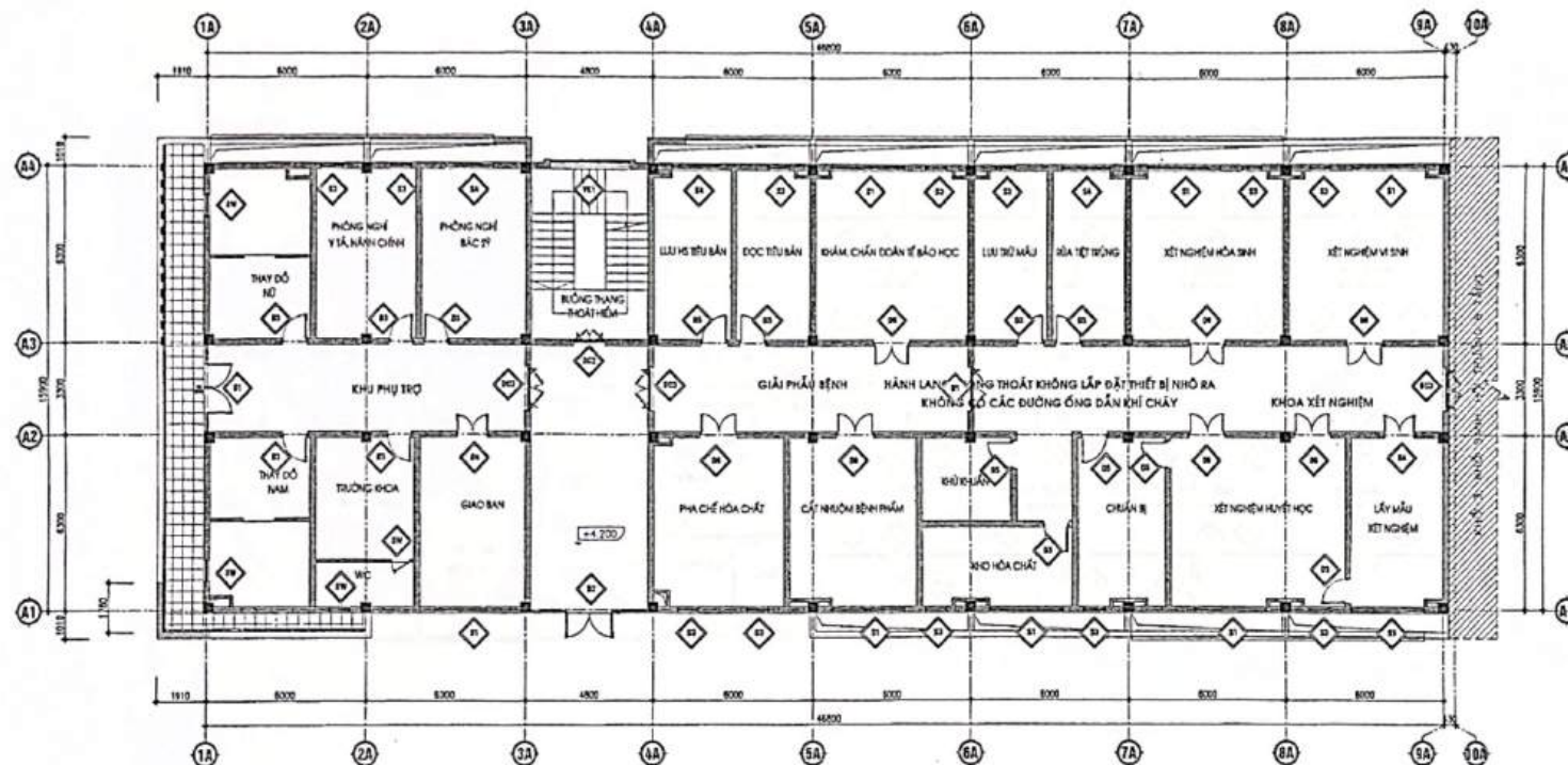
MẶT BẰNG ĐỊNH VỊ CỦA TẦNG 2
