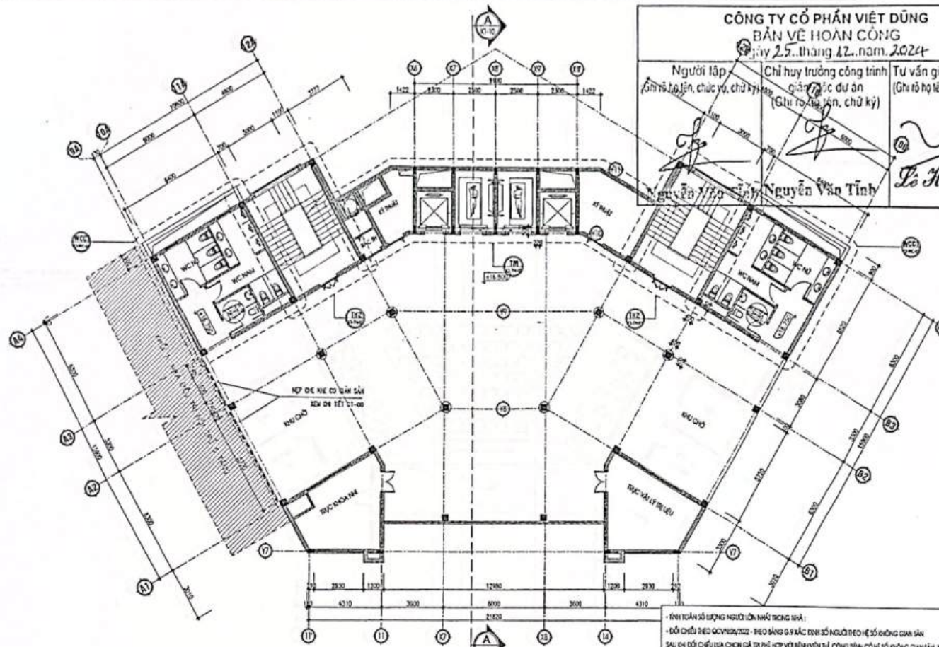
MẶT BẰNG KIẾN TRÚC TẦNG 5
