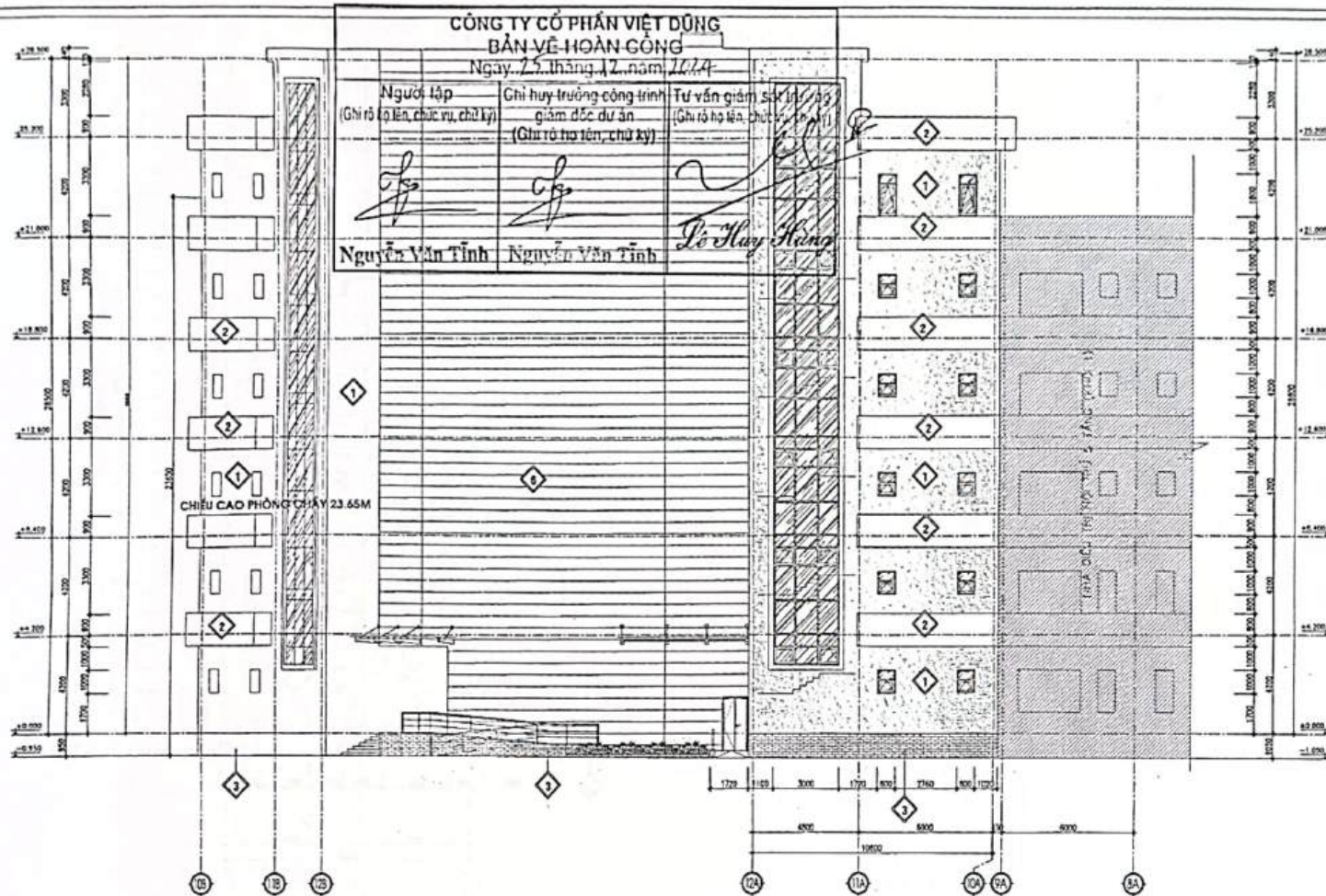
MẶT ĐỨNG TRỤC 12A-10A
