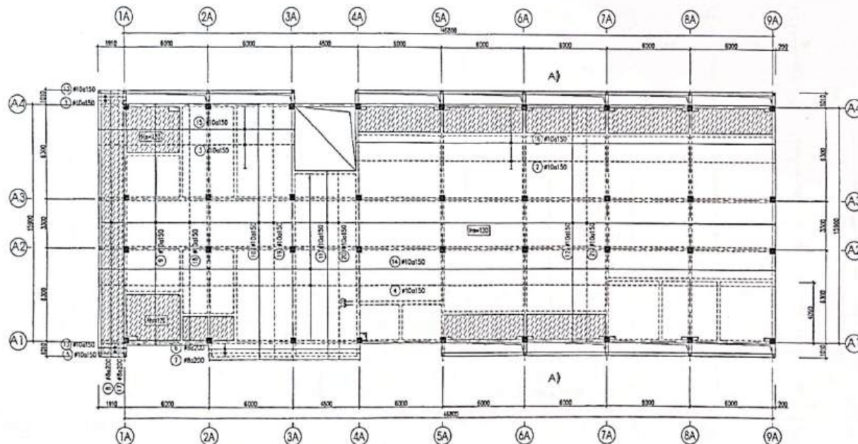
MẶT BẰNG BỐ TRÍ THÉP SÀN TẦNG 4
