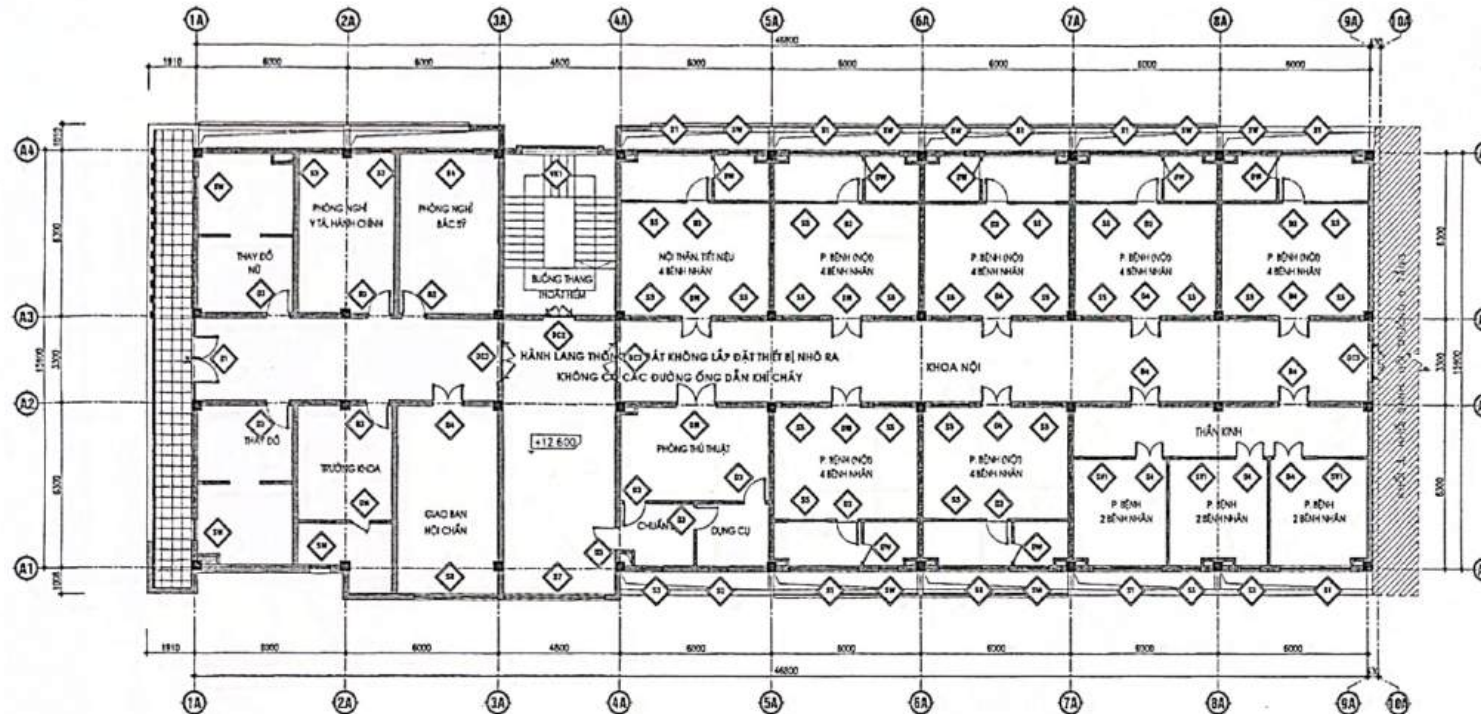
MẶT BẰNG ĐỊNH VỊ CỦA TẦNG 4
