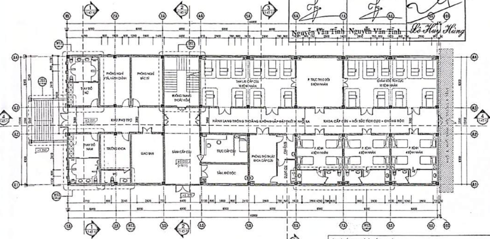
MẶT BẰNG KIẾN TRÚC TẦNG 1
