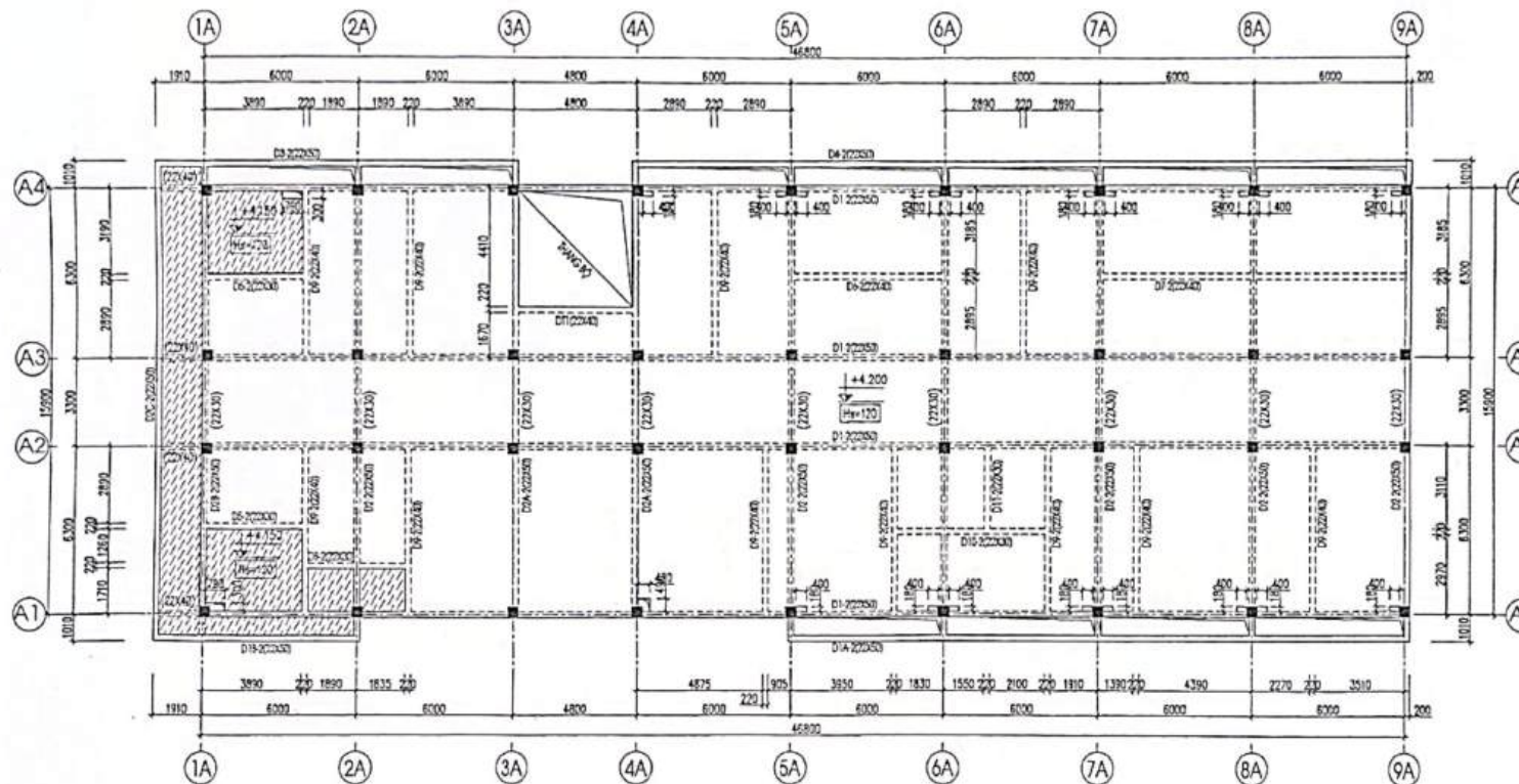
MẶT BẰNG KẾT CẤU TẦNG 2
