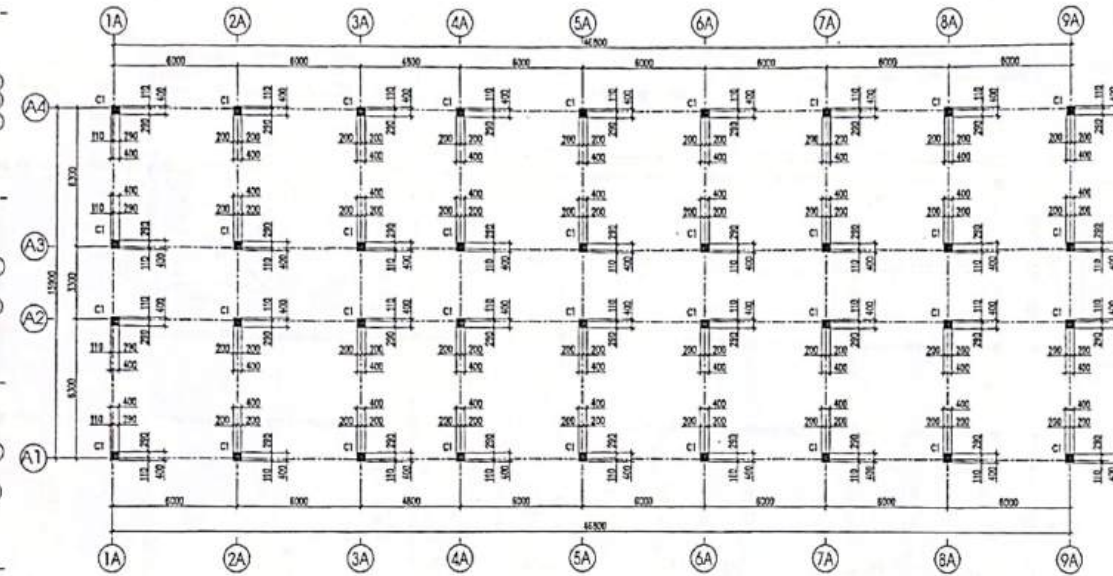
MẶT BẰNG ĐỊNH VỊ CỘT
