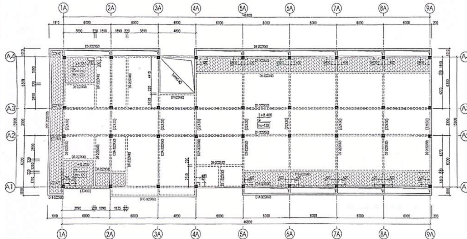
MẶT BẰNG KẾT CẤU TẦNG 3
