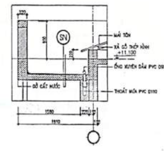
CHI TIẾT SÊ NÔ SN2
