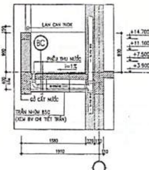
CHI TIẾT CT2
