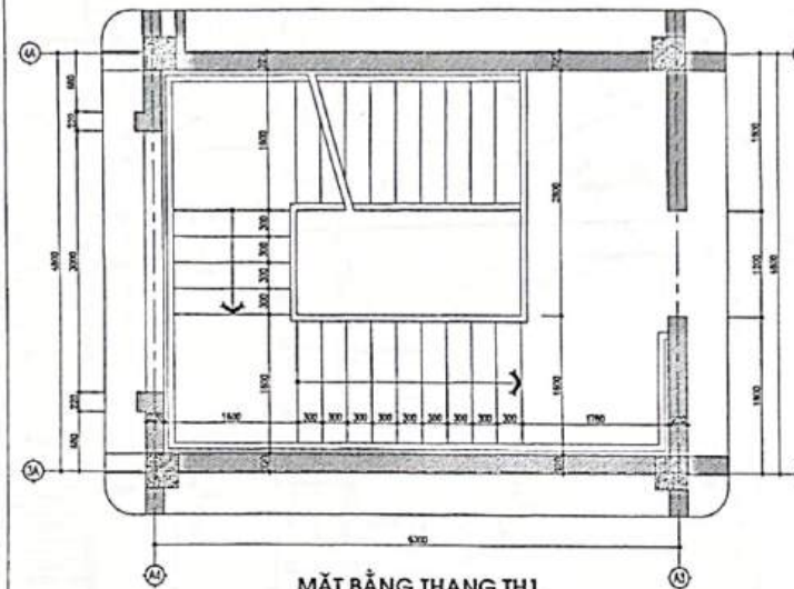
MẶT BẰNG THANG TH1 VỊ TRÍ THẺ HẸN TẦNG 5
