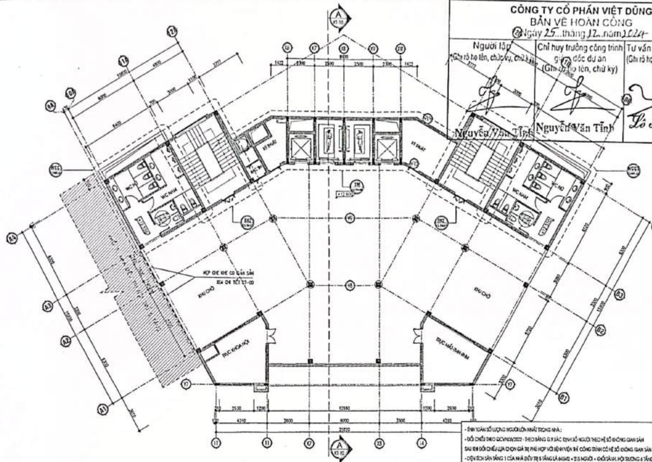
MẶT BẰNG KIẾN TRÚC TẦNG 4
