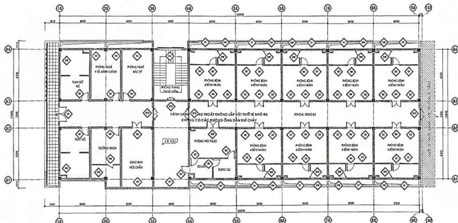
MẶT BẰNG ĐỊNH VỊ CỬA TẦNG 3
