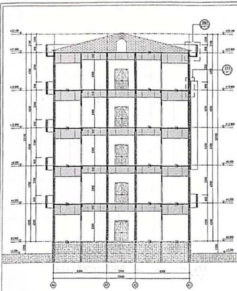
MẶT CẮT 1-1
