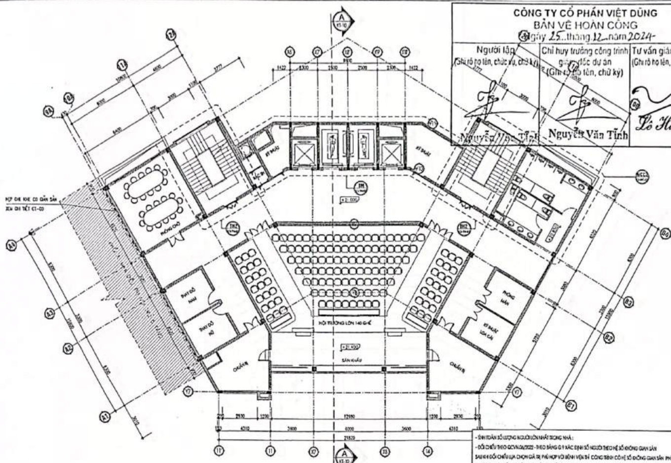
MẶT BẰNG KIẾN TRÚC TẦNG 6
