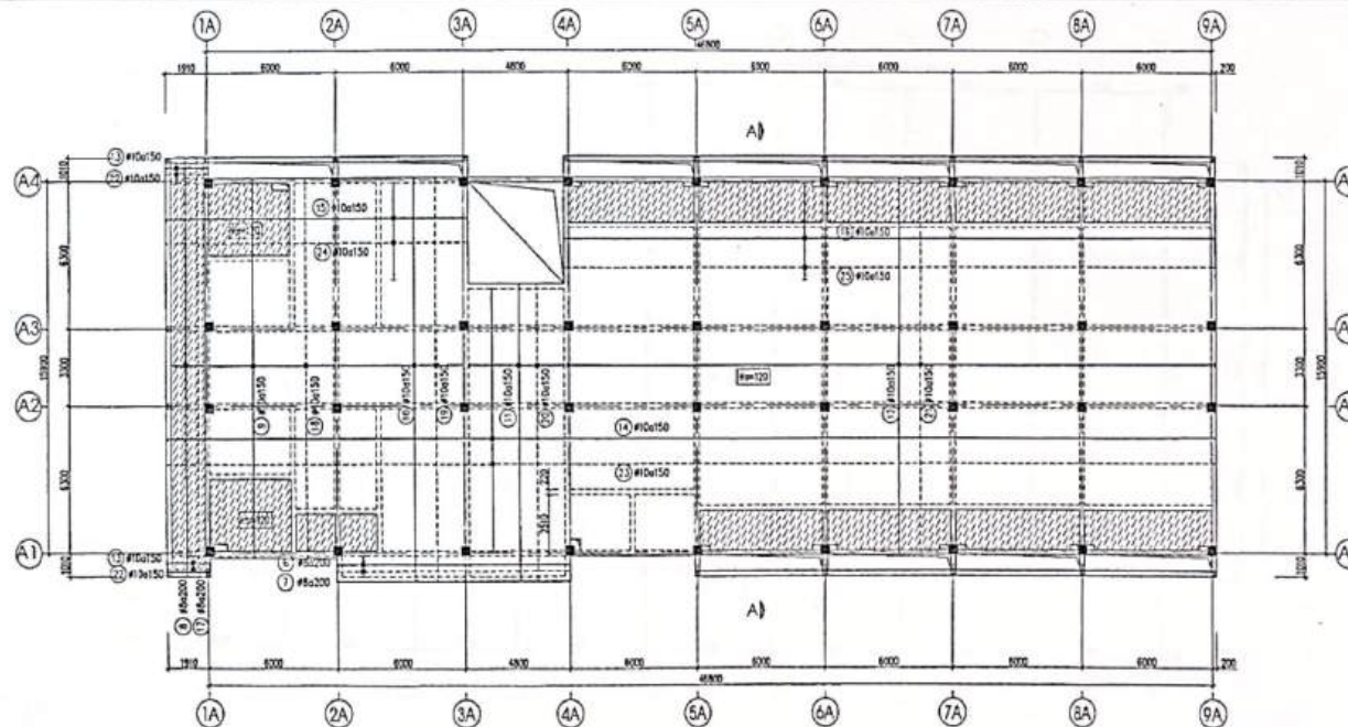
MẶT BẰNG BỐ TRÍ THÉP SÀN TẦNG 3
