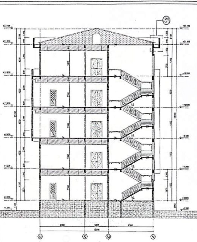
MẶT CẮT 2-2
