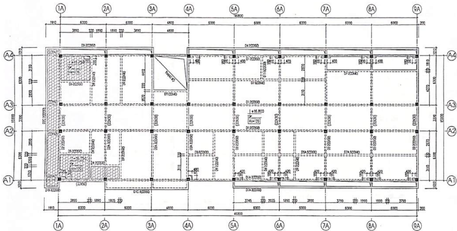
MẶT BẰNG KẾT CẤU TẦNG 5
