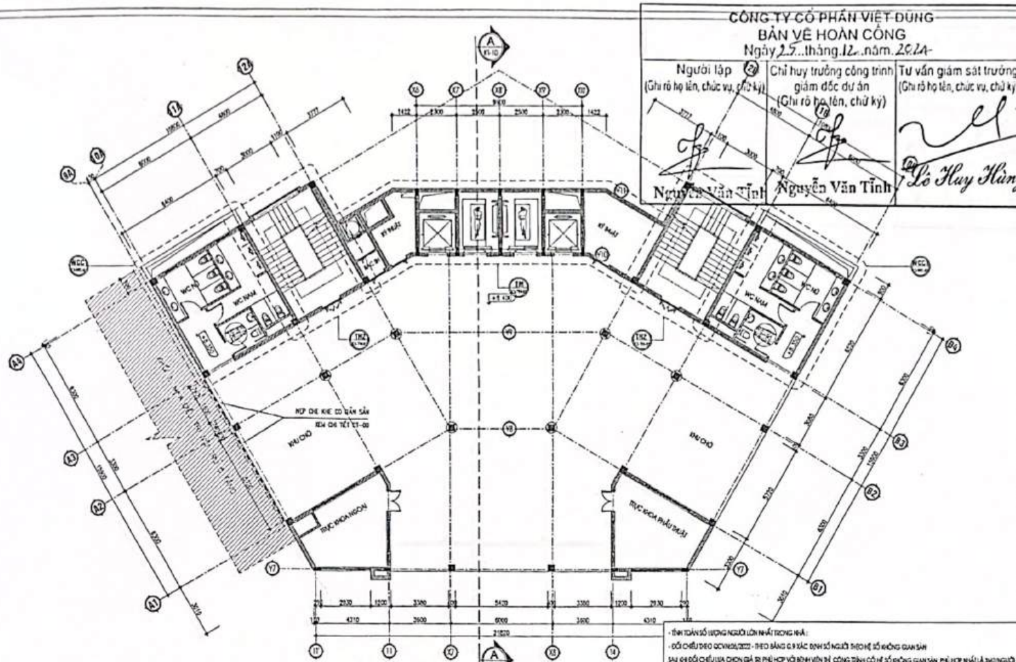
MẶT BẰNG KIẾN TRÚC TẦNG 3
