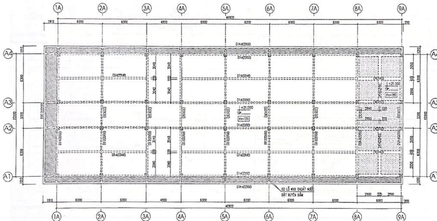
MẶT BẰNG KẾT CẤU TẦNG MÁI
