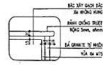
CHI TIẾT MŨI BẠC
