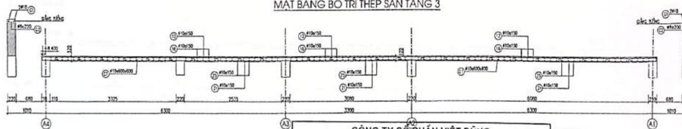
MẶT BẰNG BỐ TRÍ THÉP SÀN TẦNG 3
