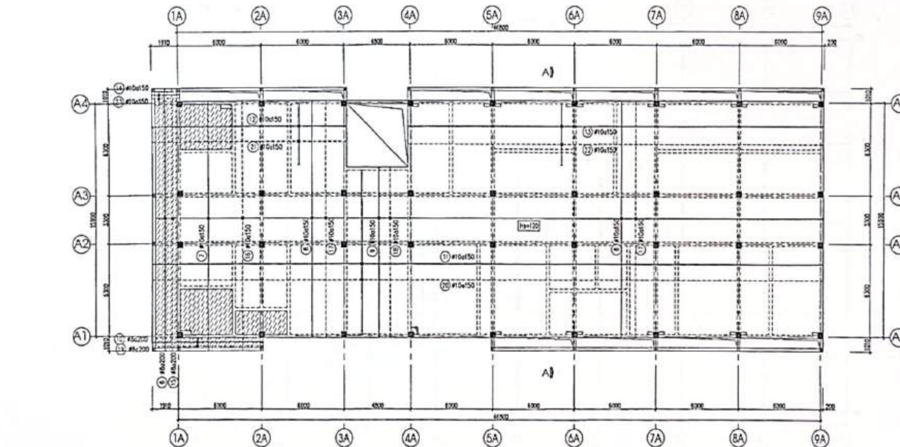
MẶT BẰNG BỐ TRÍ THÉP SÀN TẦNG 2
