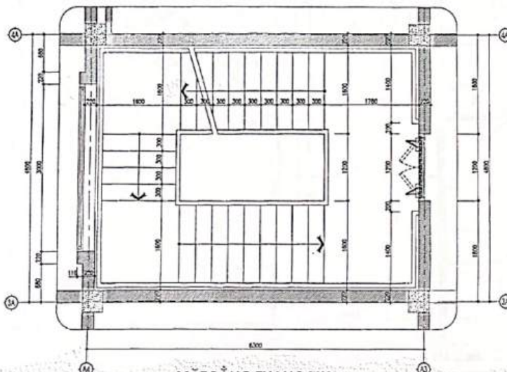
MẶT BẰNG THANG TH1 VỊ TRÍ THẺ HẸN TẦNG 2.3.4
