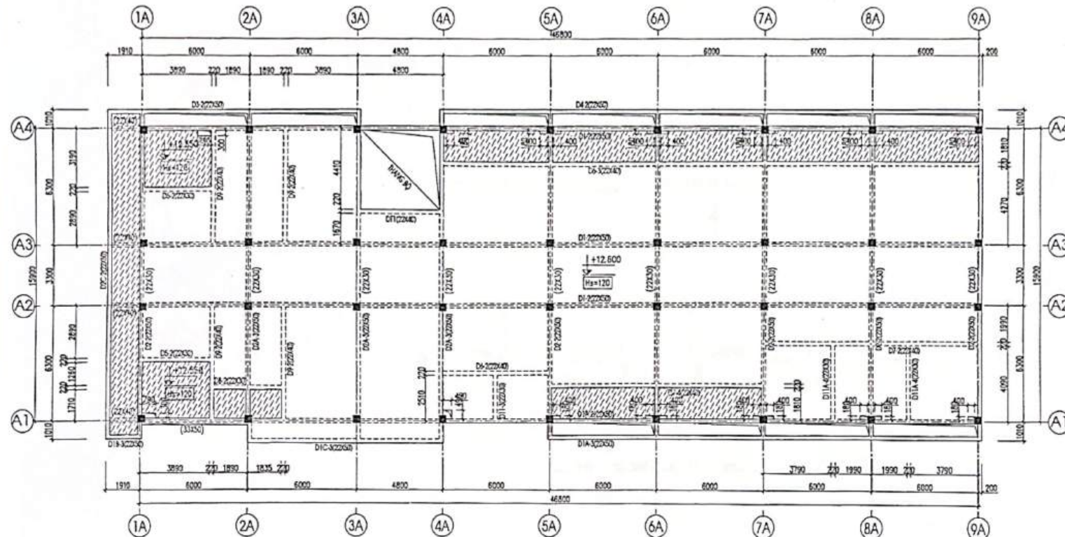
MẶT BẰNG KẾT CẤU TẦNG 4
