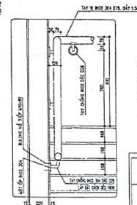
CHI TIẾT TAY VÍN
