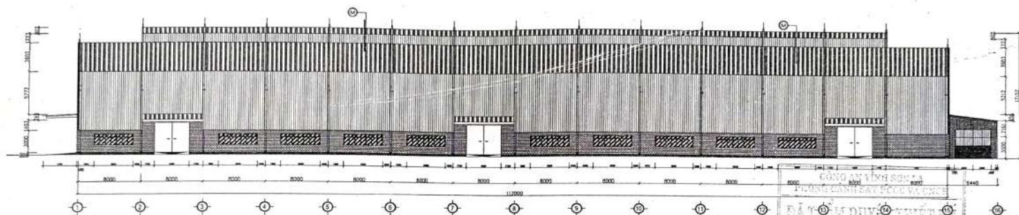
MẶT ĐÚNG TRỰC 1-15
