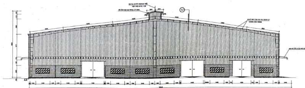
MẶT ĐỨNG TRỰC A-L
