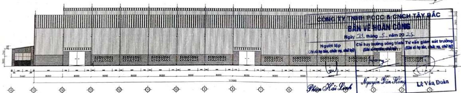
MẶT ĐÚNG TRỰC 15-1
