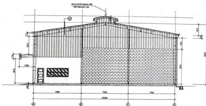
MẶT ĐÚNG TRỤC A - D
