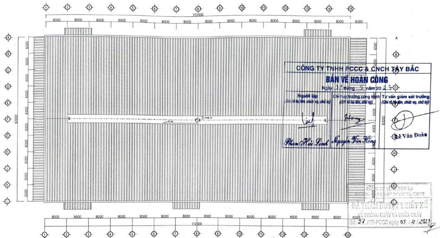
MẶT BẰNG CẢI TẠO HỆ THỐNG CHỮA BẢO TỰ ĐỘNG NHÀ XƯỞNG 01 2/2
