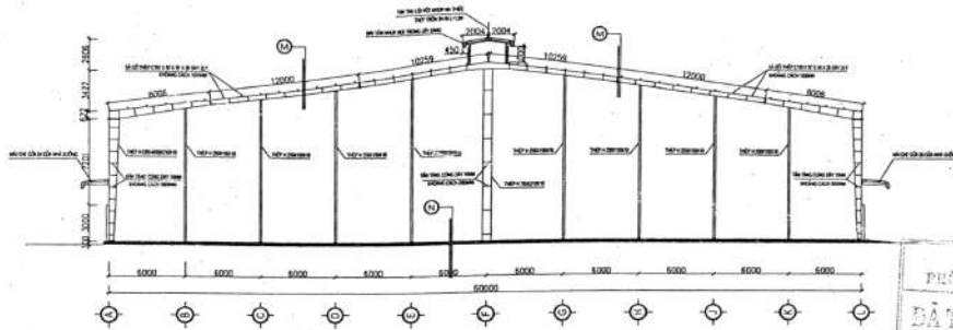
MẶT CẮT 1-1
