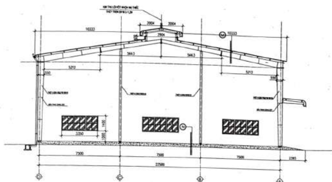
MẶT CẮT 1-1
