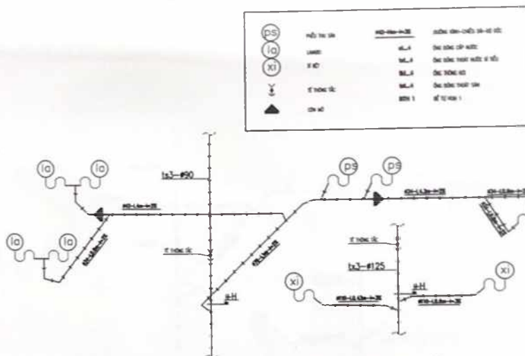
SƠ ĐỒ KHÔNG GIAN THOÁT NƯỚC TRỰC TS3, TX3 TẦNG 2,3,4,5( NHÀ B )
