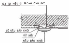
LẮP ĐẶT ĐẦU BÁO KHÓI
