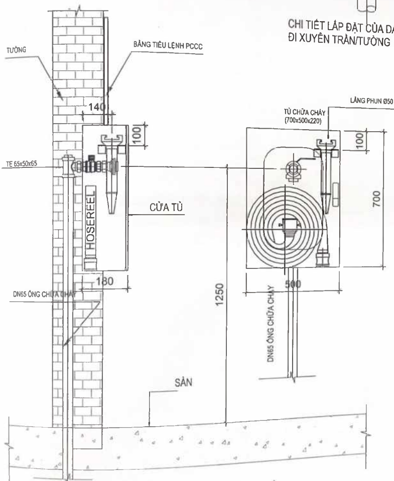
CHI TIẾT LẮP ĐẶT TỦ CHỮA CHÁY TRONG NHÀ
