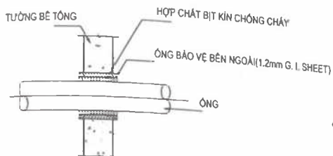
CHI TIẾT LẮP ĐẶT CỦA DẠNG ỚNG ĐI XUYÊN TRẦN/TƯỜNG
