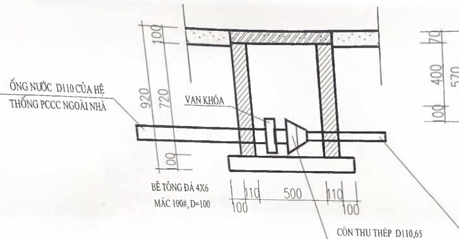
CHI TIẾT HỖ VAN NƯỚC CÓ SẴN
