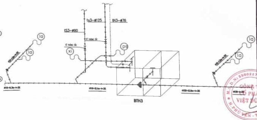
SƠ ĐỒ KHÔNG GIAN THOÁT NƯỚC TRỰC TS3, TX3 TẦNG 1 ( NHÀ B )
