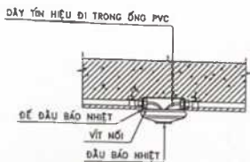
LẮP ĐẶT ĐẦU BÁO NHIỆT
