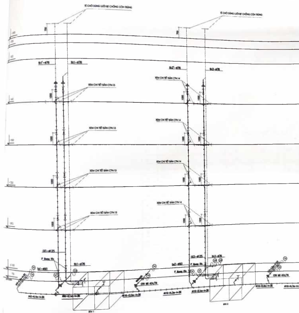
SƠ ĐỒ KHÔNG GIAN THOÁT NƯỚC TOÀN NHÀ
