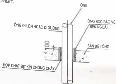
CHI TIẾT LẮP ĐẶT CỦA DẠNG ỚNG ĐI XUYÊN TRẦN/TƯỜNG
