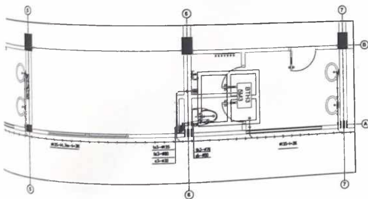
MẶT BẰNG THOÁT NƯỚC TRỤC T53, TX3 TẦNG 1 ( NHÀ B )
