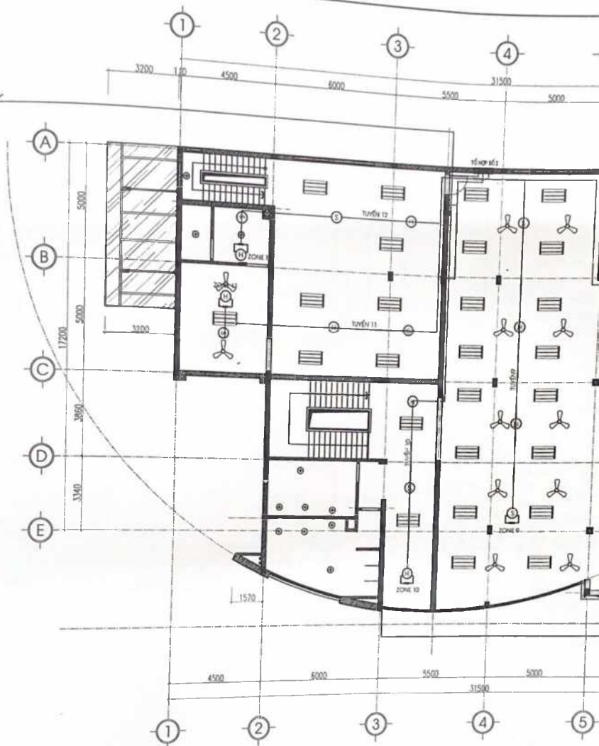
MẶT BẰNG BÁO CHÁY TẦNG 2
