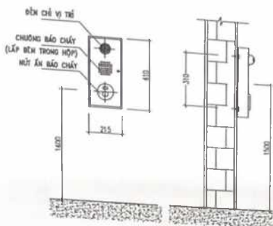
LẮP ĐẶT HỘP BÁO CHÁY TỔ HỢP
