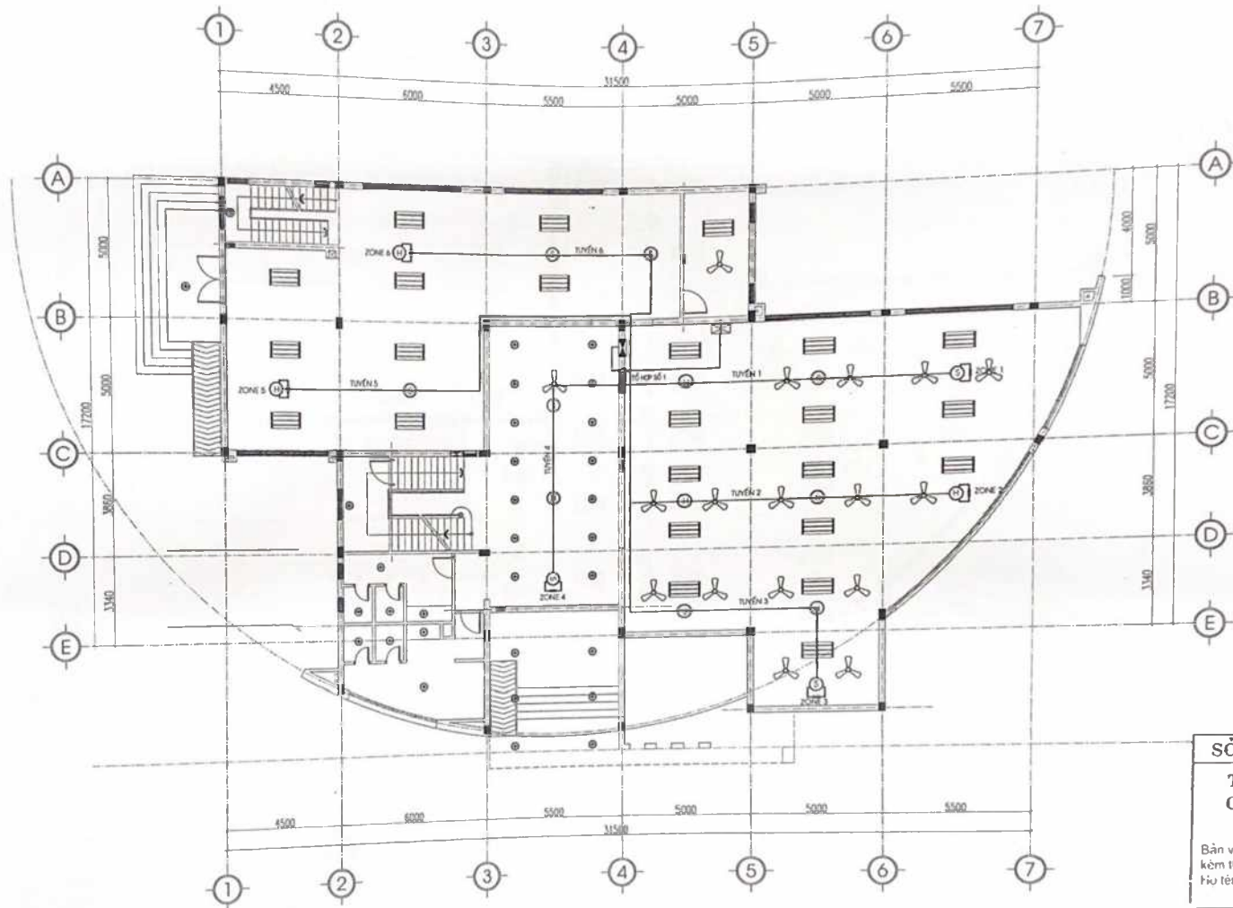
MẶT BẰNG BÁO CHÁY TẦNG 1
