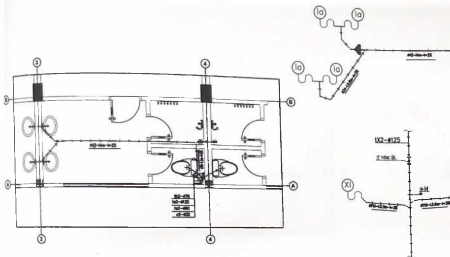
MẶT BẰNG THOÁT NƯỚC TRỰC TS2, TX2 TẦNG 2,3,4,5( NHÀ B )
