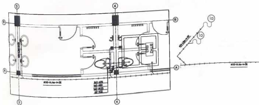
MẶT BẰNG THOÁT NƯỚC TRỰC TS2, TX2 TẦNG 1( NHÀ B )
