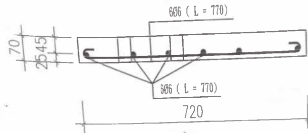
CHI TIẾT TÂM ĐAN
