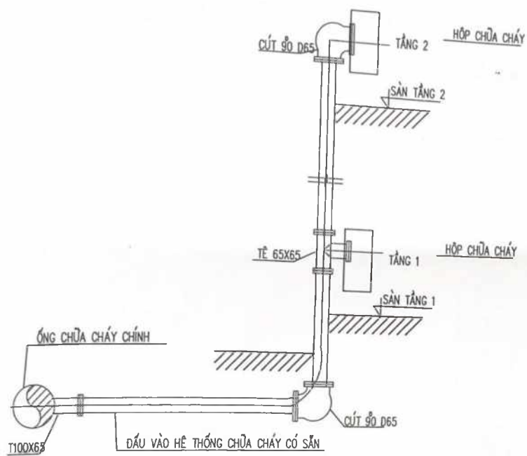
NHÁNH NƯỚC CHỮA CHÁY VÀO NHÀ
