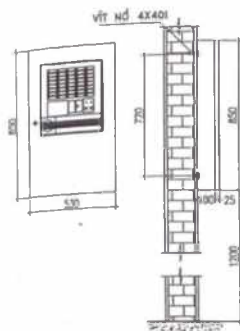
LẮP ĐẶT TRUNG TÂM BÁO CHÁY
