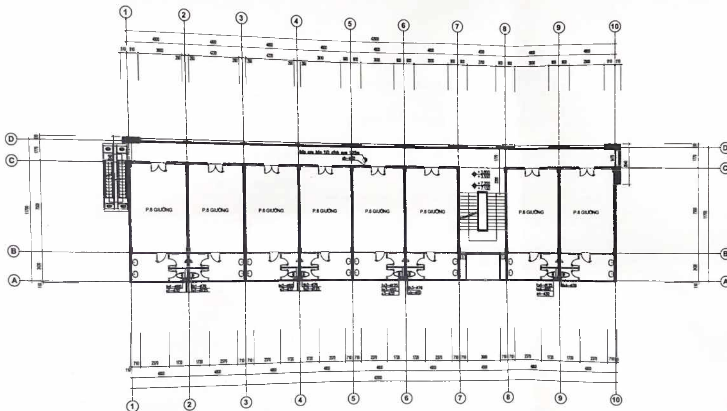
MẶT BẰNG CẤP NƯỚC CỨU HOẢ TẦNG 2,3,4,5 ( NHÀ B )
