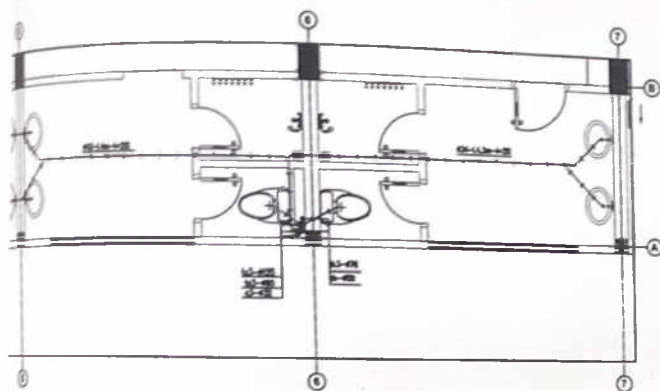
MẶT BẰNG THOÁT NƯỚC TRỰC T53,TX3 TẦNG 2,3,4,5( NHÀ B )
