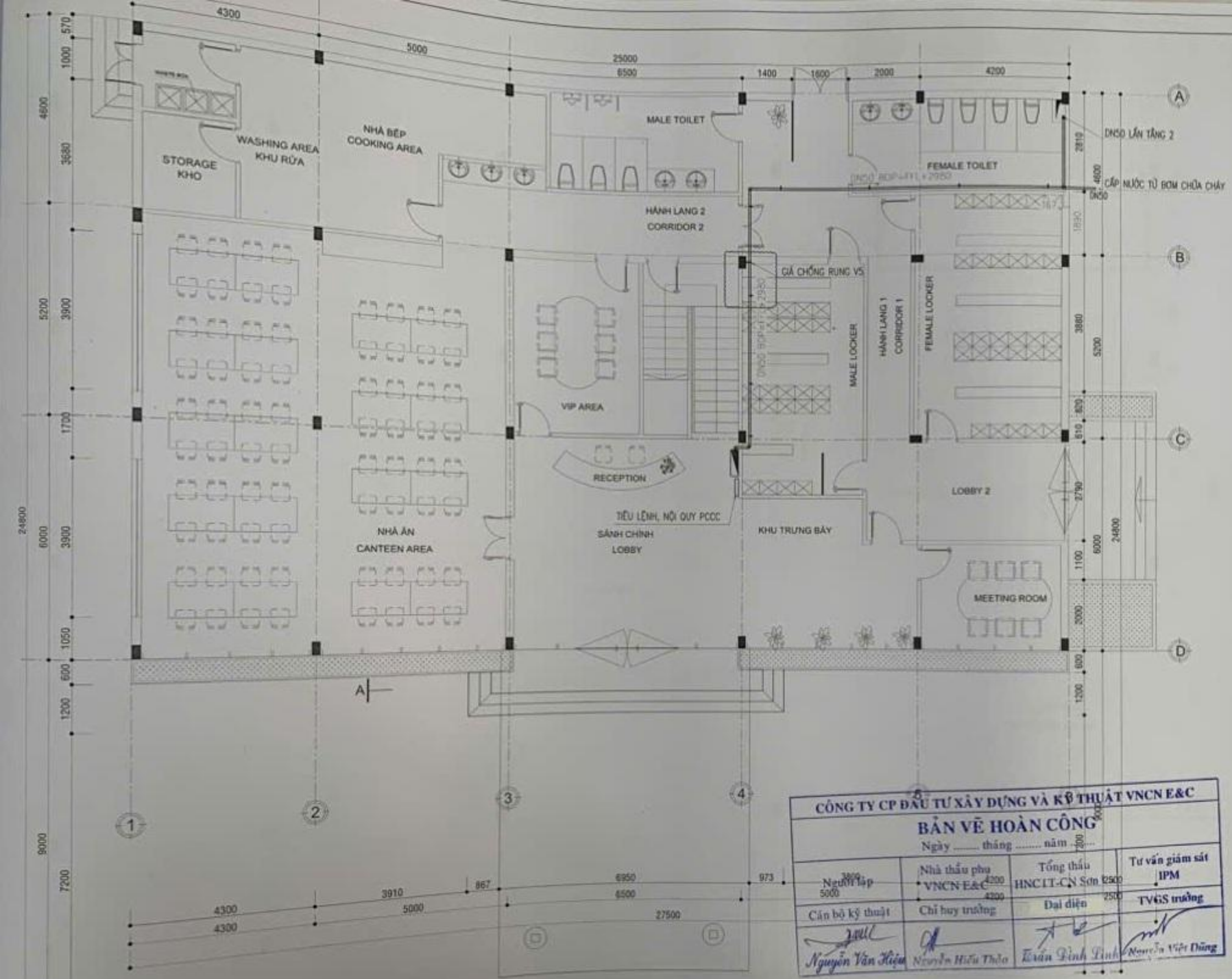
MẶT BẰNG CHỮA CHÁY TẦNG 1 NHÀ VP
