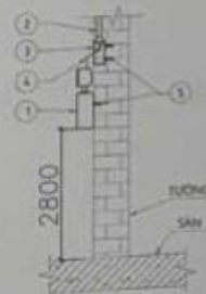
MẶT CẠNH/SIDE VIEW
